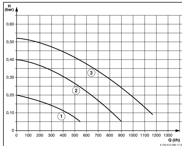
Рис 36 Характеристики насосов при ZWC 24-3, ZSC 24-3 (без монтажной присоединительной панели)
