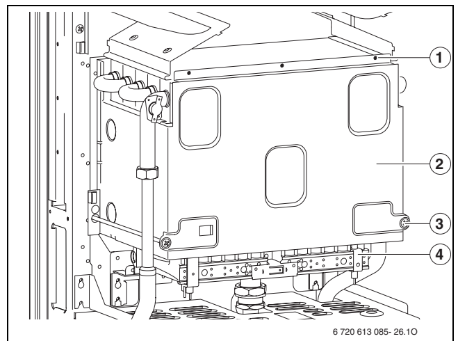
Рис 49 Открытие горелки
